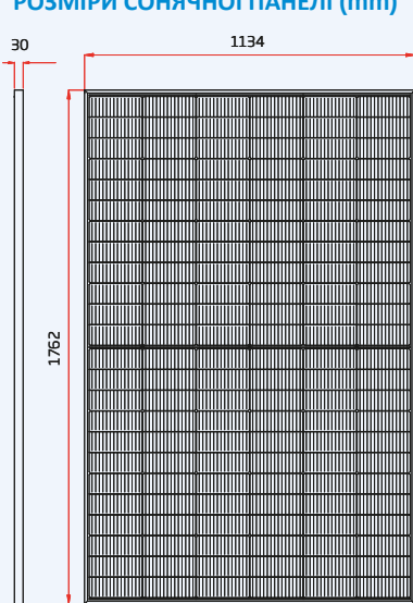
Вигляд спереду
